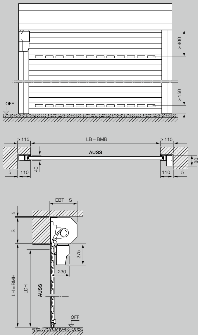
Dimensiuni pentru uși-rulou interioare și exterioare
