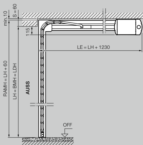
Gamă de dimensiuni ușă cu șină de rulare la tavan RollMatic OD*
